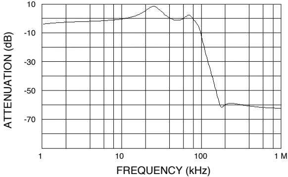
FMCE-0328 Attenuation
